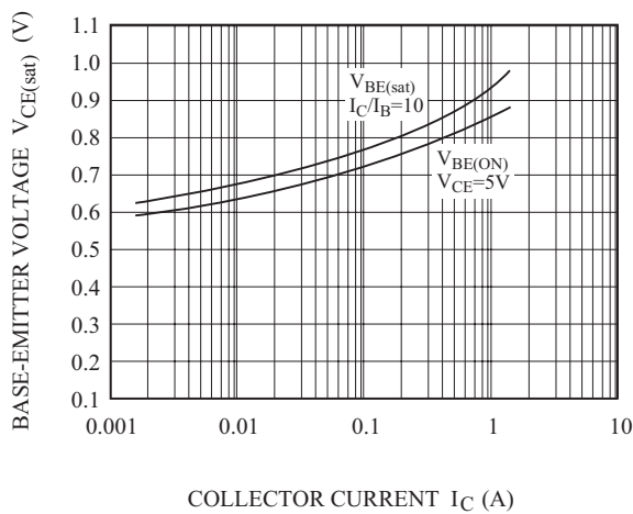
V_{CE(sat)} - I_C
