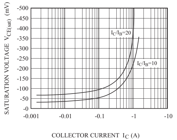
V_{CE(sat)} - I_C
