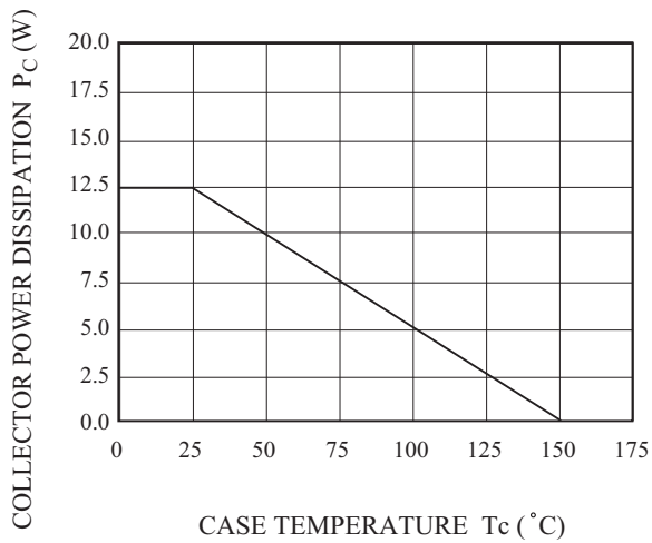
P_C - T_C
