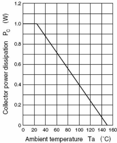
P_C - T_a
