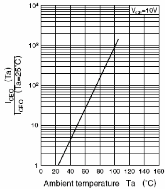
I_{CEO} - T_a
