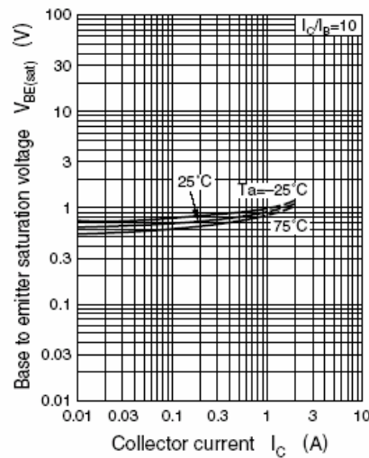
V_{BE(sat)} - I_C
