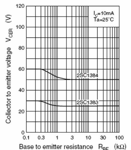
V_{CER} - R_{BE}
