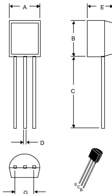
DIMENSIONS
