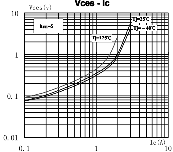
V_{ces} - I_c
