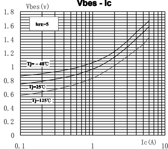
V_{bes} - I_c
