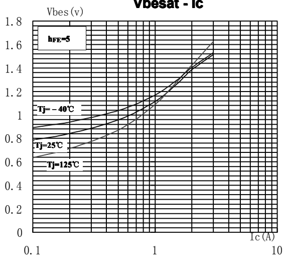
V_{besat} - I_c
