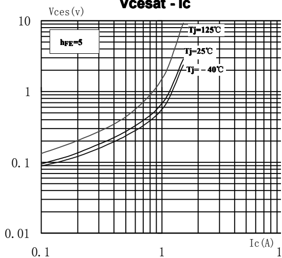
V_{cesat} - I_c
