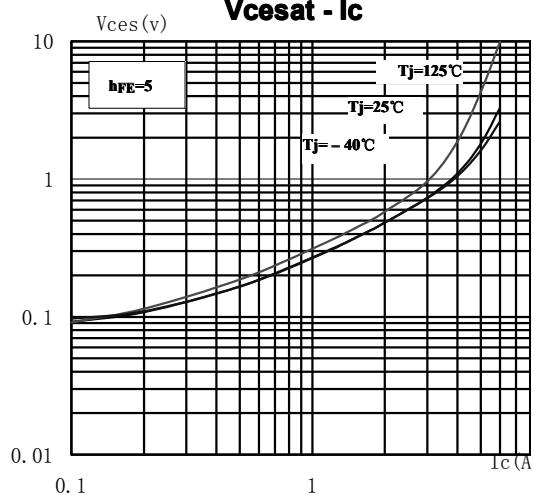
V_{cesat} - I_c
