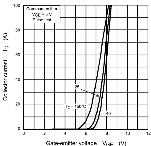
Fig. 8.5 I_c - V_{ge}
