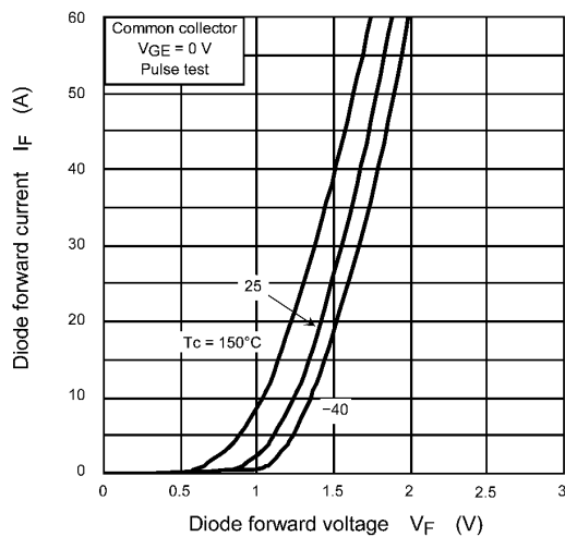
Fig. 8.13 I_F - V_F
