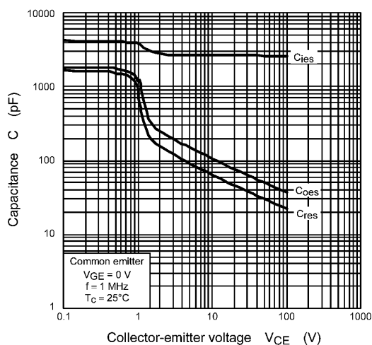
Fig. 8.7 C - V_{CE}
