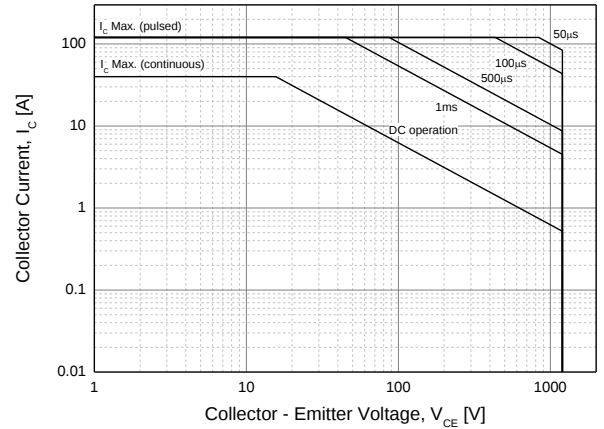
Fig. 14 SOA
