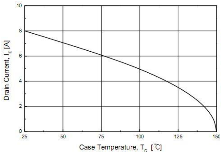
TMP8N80(G)
