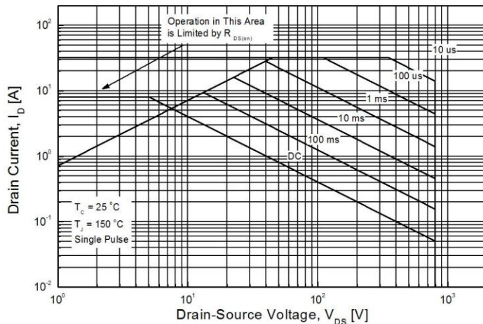
TMPF8N80(G)
