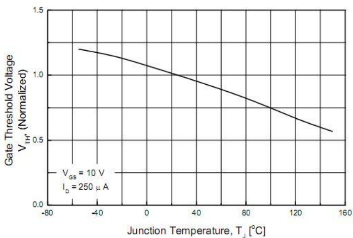
TMPF8N80(G)
