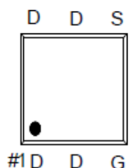
PDFN 2X2S
