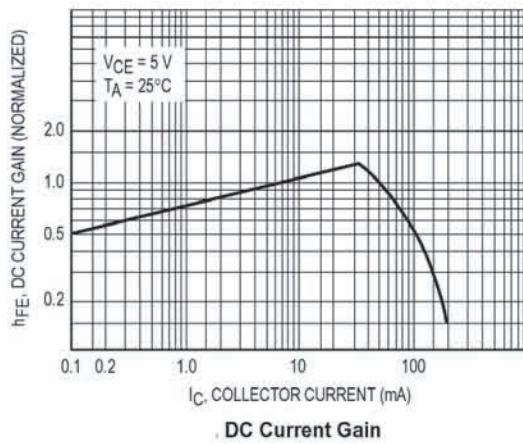
BC547/BC548
